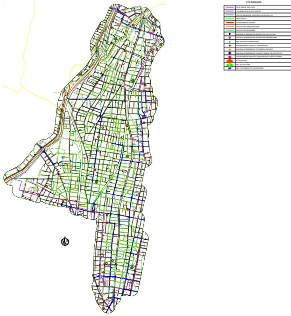
Εικόνα 8.: Γενική Διάταξη Έργων Πιεζομετρικής Ζώνης PRV Δεξαμενής Χολαργού
