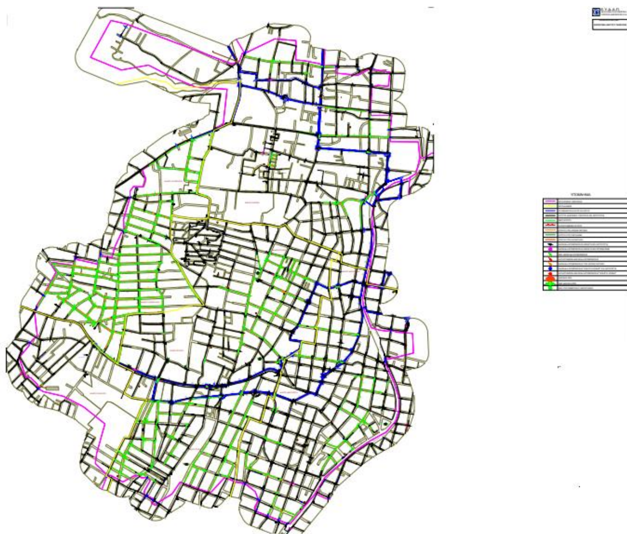
Εικόνα 10.: Γενική Διάταξη Έργων Πιεζομετρικής Ζώνης PRV Μπότσαρη και Κοκκινάκη
