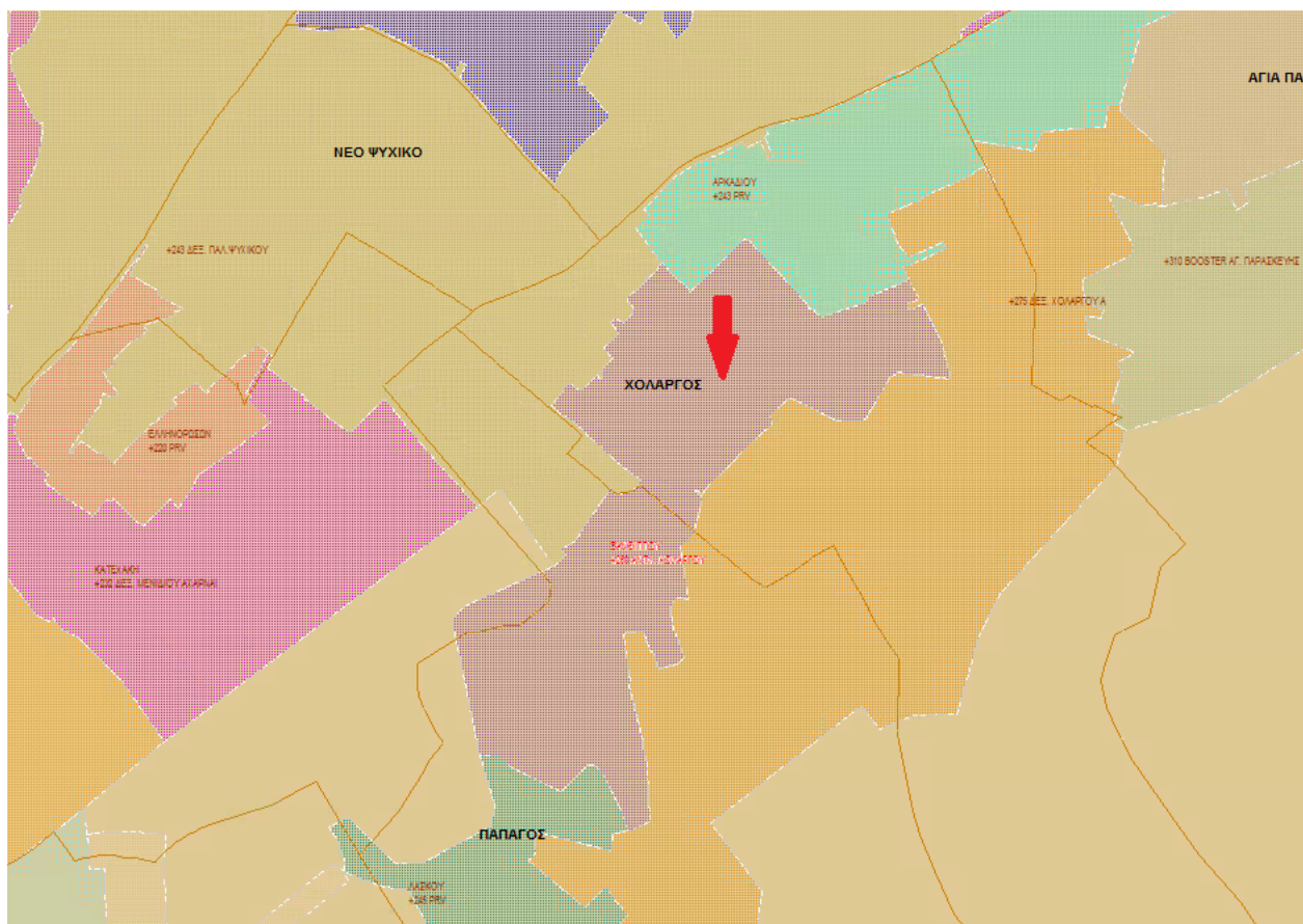
Εικόνα 5.: Χαρτογραφική απεικόνιση της ζώνης υδροδότησης Ξανθίππου Αντλιοστάσιο Χολαργού +260PRV
