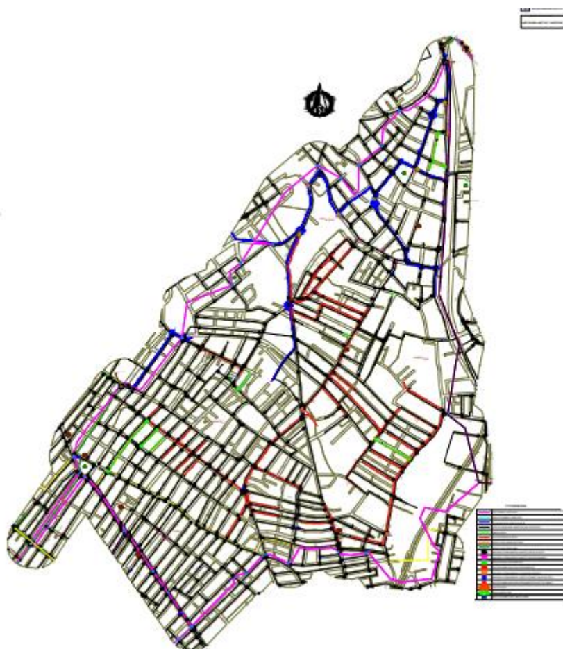
Εικόνα 14.: Γενική Διάταξη Έργων Πιεζομετρικής ζώνης PRV Αργυροκάστρου
